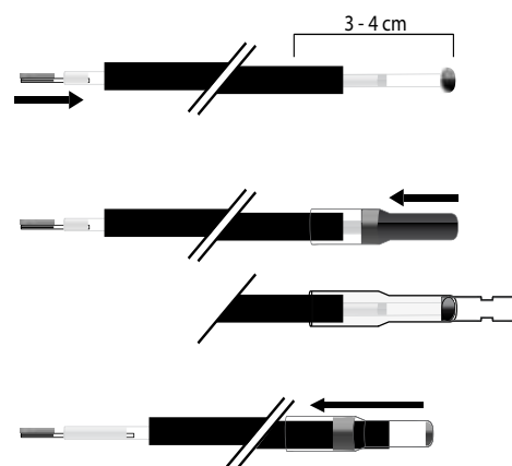
Ensamble de la sonda, conductor y tapa metálica
